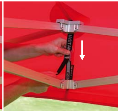
SCHRITT 10 ZIEHEN SIE DIE LASCHE SOWEIT NACH UNTEN, BIS DAS ZELTDACH VOLLSTÄNDIG AUFGESpanNT IST.
