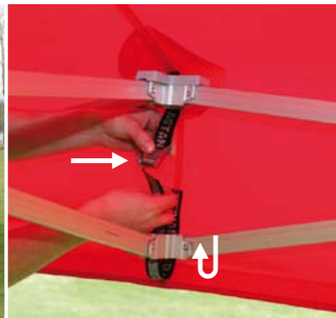
SCHRITT 9 FÜHREN SIE DIE LASCHE DURCH DIE VERBINDER UND SCHNALLEN.
