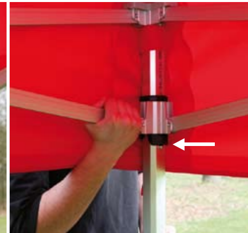
SCHRITT 6 DIE RICHTIGE POSITION IST ERREICHT, WENN DER ECK-SCHIEBER ÜBER DIE SICHERUNG GESCHOBEN IST.
